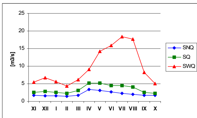
Rysunek 3. Gmina Łądek Zdrój – charakterystyczne przepływy wody rzeki Biała Łądecka ( \text{m}^3/\text{s} ) w okresie 1971 – 1990 na profilu Łądek Zdrój [SNQ – średnia niska woda; SQ – średnia roczna woda; SWQ – średnia wielka woda; profil Łądek Zdrój – 420,52 m n.p.m., km biegu rzeki 22,4; źródło: Komentarz do Mapy Hydrograficznej w skali 1:50000, arkusz M-33-58-D, Złoty Stok (Baraniecki, Bieroński, Pawlak, Tomaszewski, 1998)]
