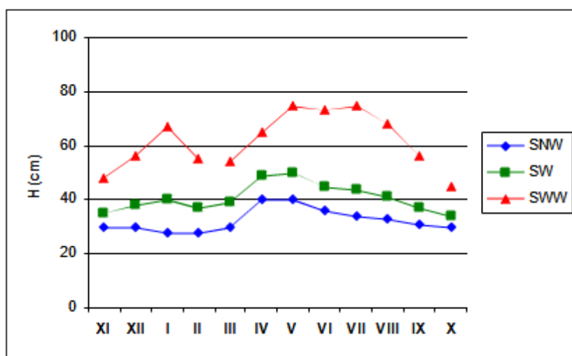
Rysunek 2. Gmina Łądek Zdrój – charakterystyczne miesięczne stany wody rzeki Białej Łądeckiej (cm) w okresie 1951 – 1990 na profilu Łądek Zdrój [SNW – średnia niska woda; SW – średnia roczna woda; SWW – średnia wielka woda; profil Łądek Zdrój – 420,52 m n.p.m., km biegu rzeki 22,4; źródło: Komentarz do Mapy Hydrograficznej w skali 1:50000, arkusz M-33-58-D, Złoty Stok (Baraniecki, Bieroński, Pawlak, Tomaszewski, 1998)]
