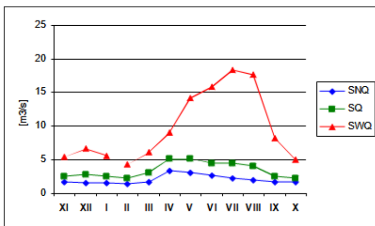
Rysunek 3. Gmina Łądek Zdrój – charakterystyczne przepływy wody rzeki Biała Łądecka ( m^3/s ) w okresie 1971 – 1990 na profilu Łądek Zdrój [SNQ – średnia niska woda; SQ – średnia roczna woda; SWQ – średnia wielka woda; profil Łądek Zdrój – 420,52 m n.p.m., km biegu rzeki 22,4; źródło: Komentarz do Mapy Hydrograficznej w skali 1:50000, arkusz M-33-58-D, Złoty Stok (Baraniecki, Bieroński, Pawlak, Tomaszewski, 1998)]
